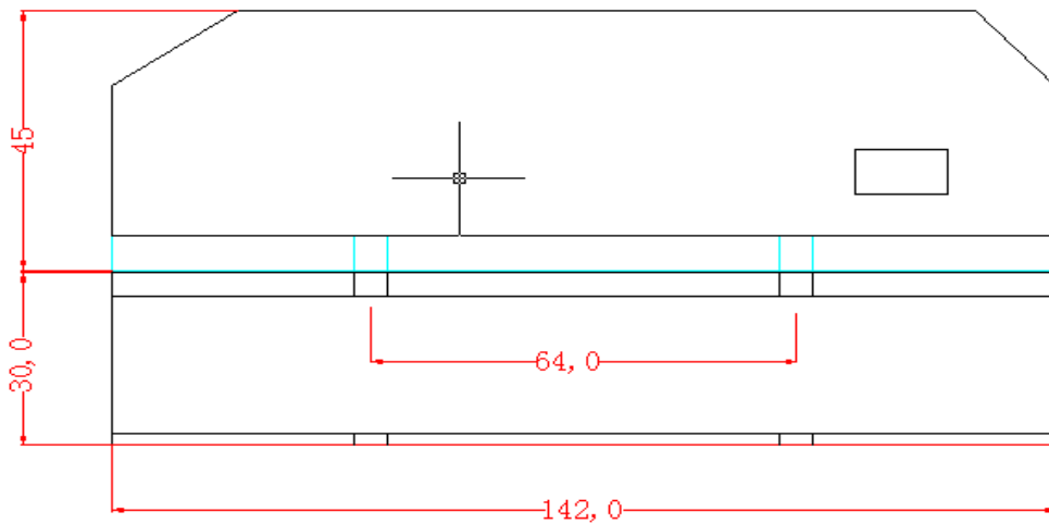
外形尺寸图
